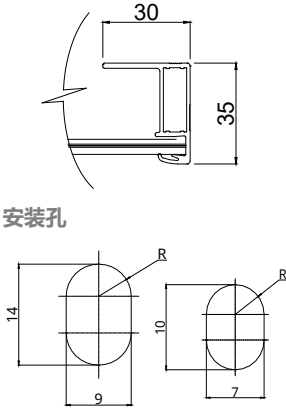
边框横截面 A-A
