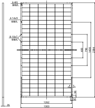
背面图
