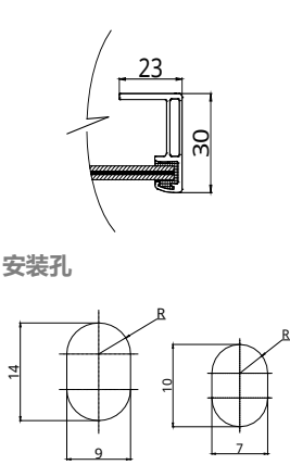
边框横截面 A-A
