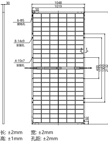
背面图
