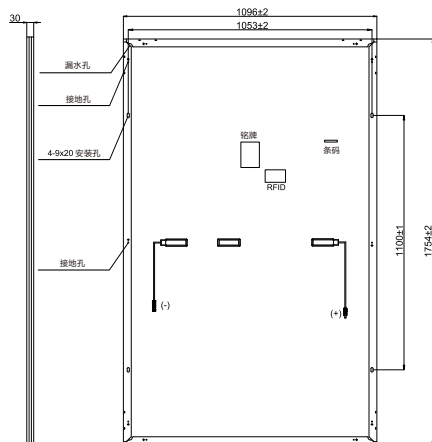
产品图示 单位: mm
