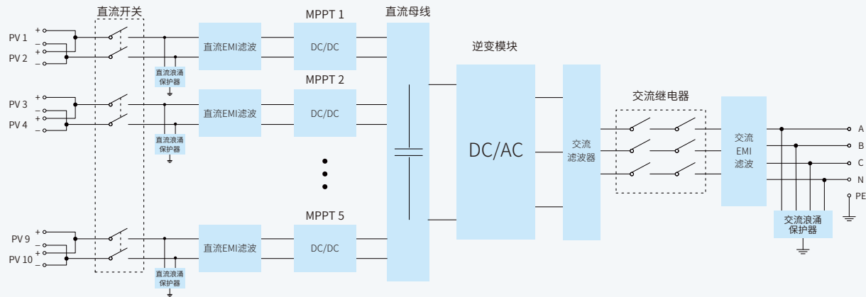
电路框图
