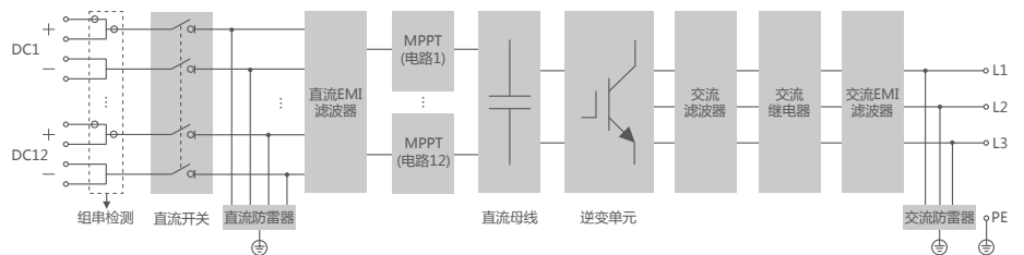
电路框图
